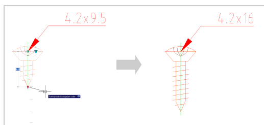
Abb. 2: Bearbeitung eines dynamischen Blocks über die Griffe
